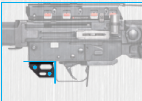
Stgw 57-Ordonnanz-Schnittstelle (Direktmontage)
