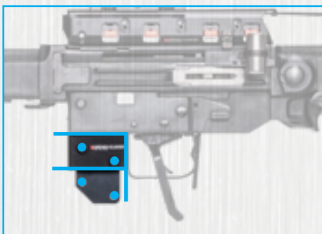
Stgw 57 mit 57er- Winterabzugadapter (Art.: 14.9818.1)
