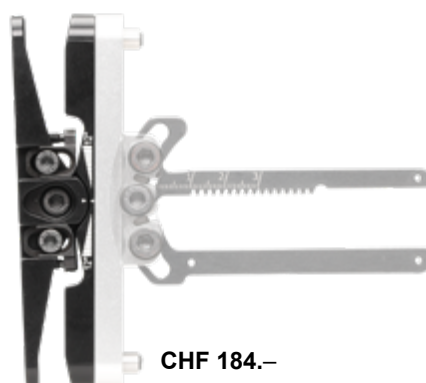
Art. Nr. 14.8129 ● Angle Plate ohne Support für Direktmontage auf bestehende Grundplatten oder Holzschäfte, 118g
