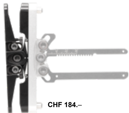
Art. Nr. 14.8129 ● Angle Plate ohne Support für Direktmontage auf bestehende Grundplatten oder Holzschäfte, 118 g
