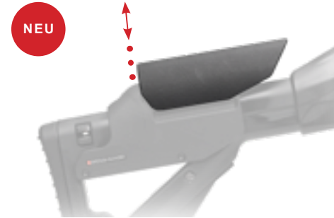
Art. Nr. 14.9747.01-14.9747.10 G+E Stgw 90 Zusatzerhöhung Schiebekolben Grössen (Höhen): 2.5/5/7.5/10/12.5/15/17.5/ 20/22.5 und 25mm
